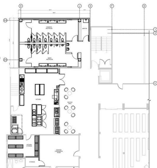
Segundo Nivel
