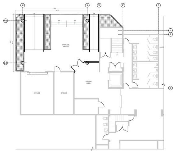
Primer Nivel
