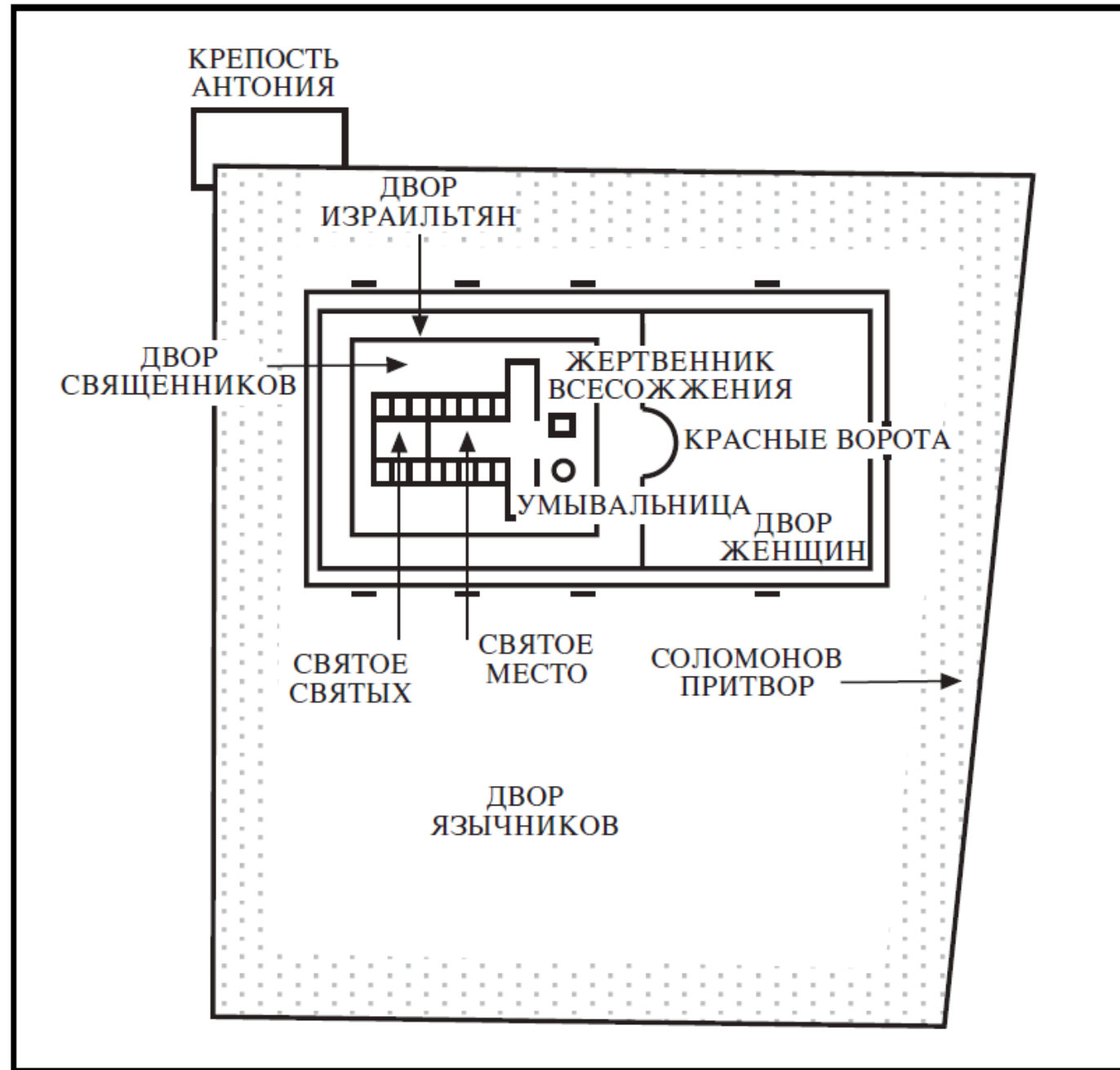
Схема храма
